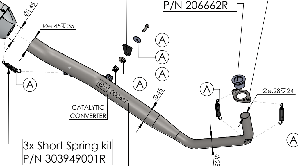
S.S. Pipe n°1471 kit P/N 3014340206R
